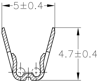
断面 B-B SECT B-B
