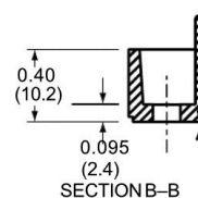
0.095 (2.4) SECTION B-B
