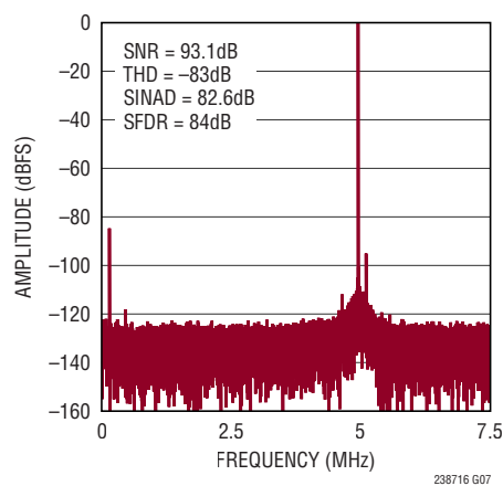
32k Point FFT f_{\text{SAMPL}} = 15\text{Mpsps} , f_{\text{IN}} = 5\text{MHz}
