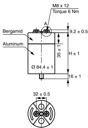
Drawing 1 i.e.: HDMKP...-...I
