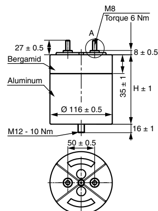
Drawing 4 i.e.: HDMKP...-...B
