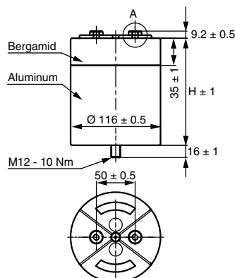
Drawing 3 i.e.: HDMKP...-...I
