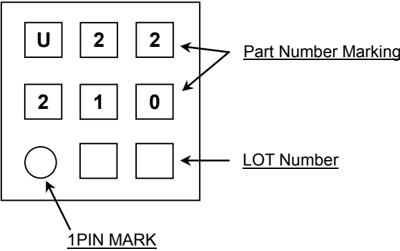
VQFN016V3030(TOP VIEW)
