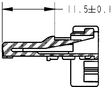
断面 A-A
