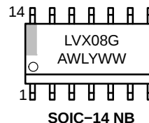
SOIC-14 NB
