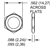
Hex Nut
