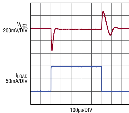
V_{CC2} Load Step (100mA)
