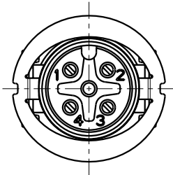
4pol A-Codierung (Steckseite) 4pole A-coding (Plug-in side)
