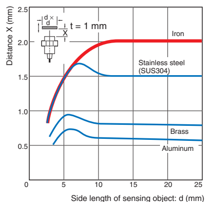
E2E-X2ME/-X2MY/-X2MF
