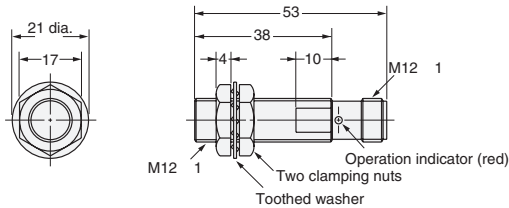
Diagram 24 E2E-X7D□-M1(G)/E2E-X5E□-M1/X5F□-M1 E2E-X5Y□-M1
