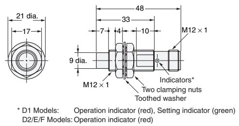
Diagram 23 E2E-X5MY□-M1
