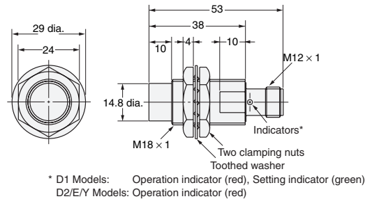
Diagram 27 E2E-X20MD□-M1(G)/E2E-X18ME□-M1/ X18MF□-M1 E2E-X18MY□-M1
