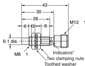
Diagram 19 E2E-X4MD□-M1(G) E2E-X2ME□-M1/E2E-X2MF□-M1
