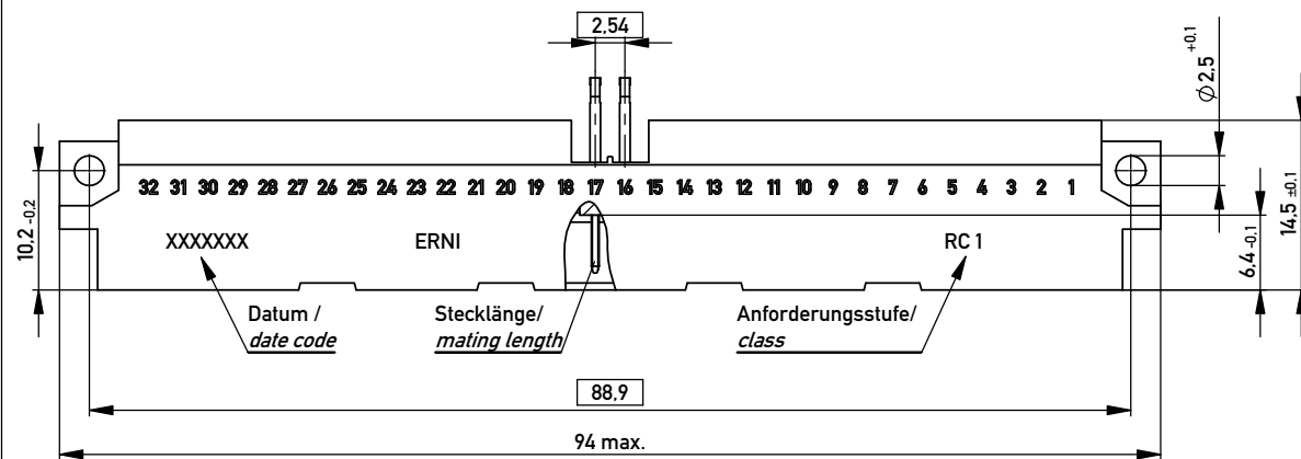
Bestückungsplan / contact layout
