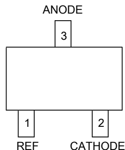
SOT23
