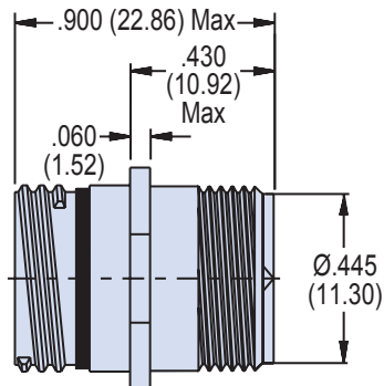
801-089-01 Inline
