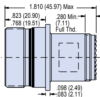
Inline Receptacle
