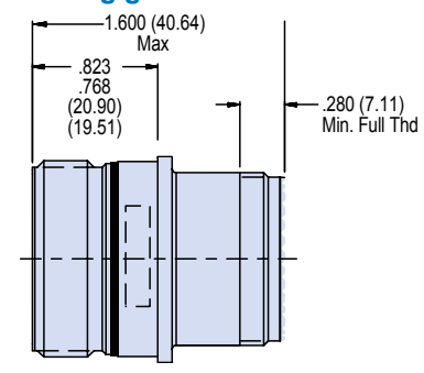
Inline Receptacle
