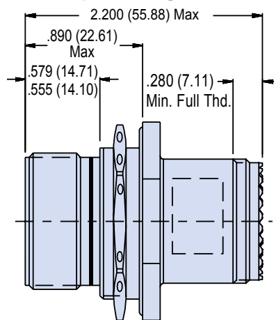
Jam Nut
