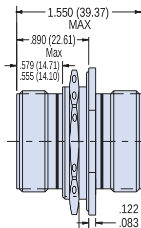
Jam Nut
