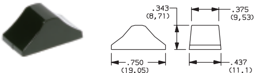
Cap, 03 actuator
