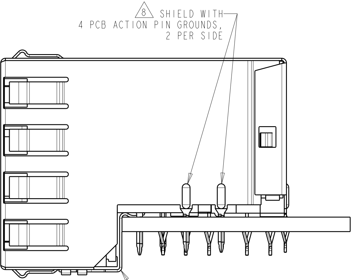
P/N 6116317-3, -9, -1/0 SCALE 4:1
