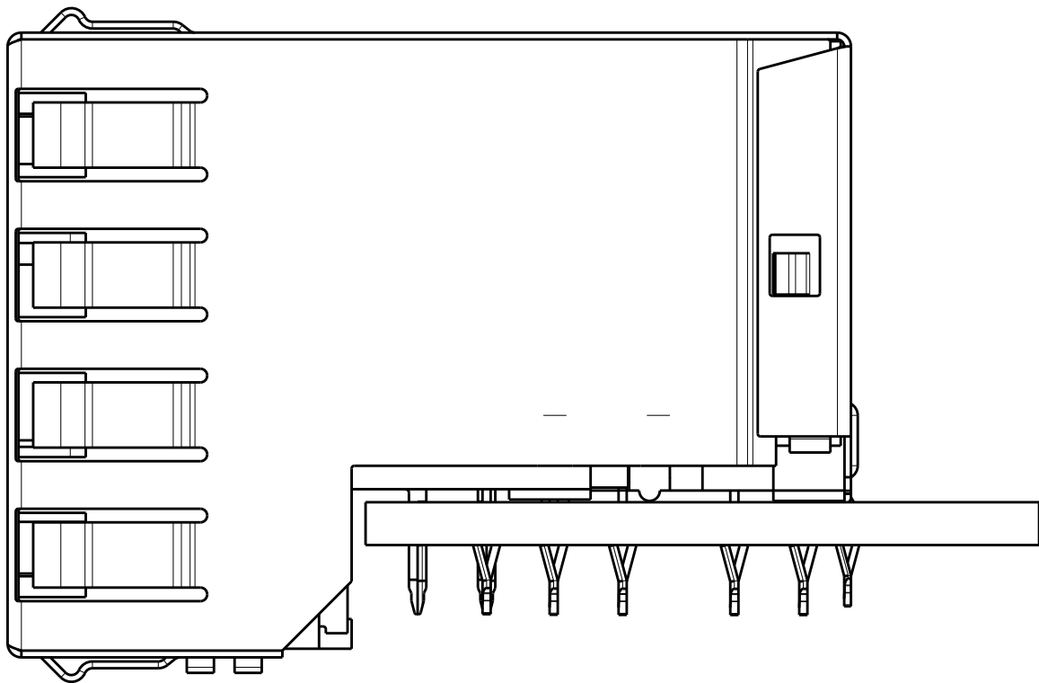
P/N 6116317-1, -8 SCALE 4:1
