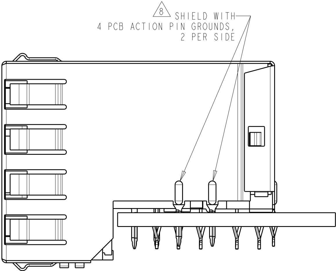
P/N 6116317-2, -5, -6, -7, SCALE 4:1
