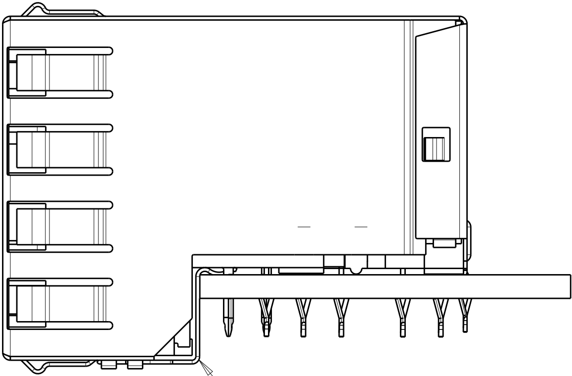
P/N 6116317-4 SCALE 4:1
