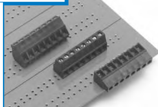
ELXM . . . . . Page 61 12A / 300V
