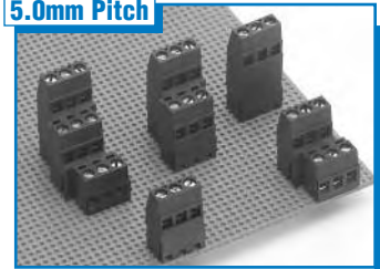
ESMT Multi-tier . . . . . Pages 70-71 17.5A / 300V
