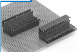
ELFD 2-Tier Offset H/V . . . . . Page 48 15A / 300V
