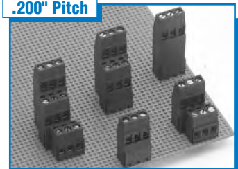
ESTT Multi-tier . . . . . Pages 72-73 24A / 300V
