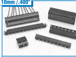
ELLP, ELLT, ELLF, ELLK . . . Page 53 15A / 600V
