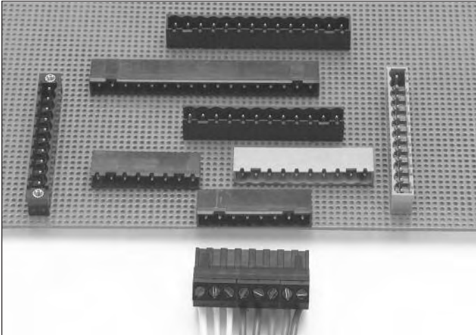
ELFH Horizontal—Eared
