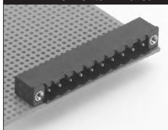
ELFH Horizontal—Eared
