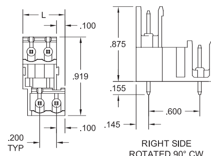
ELFD—Vertical
