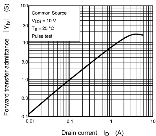
Fig. 7.8 |Y_{fs}| - I_D
