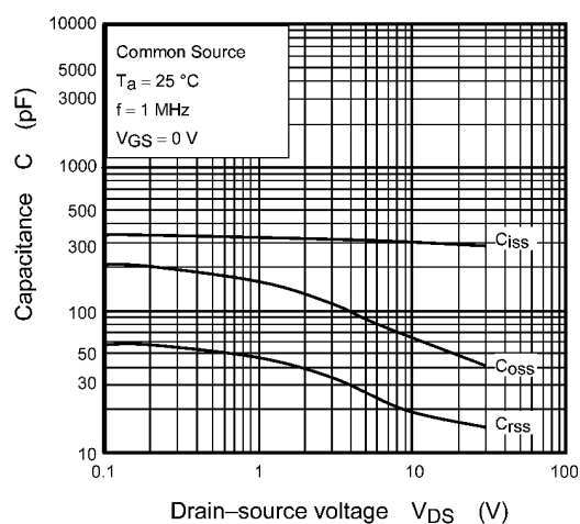
Fig. 7.10 C - V_{DS}
