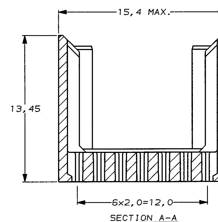
SECTION A-A
