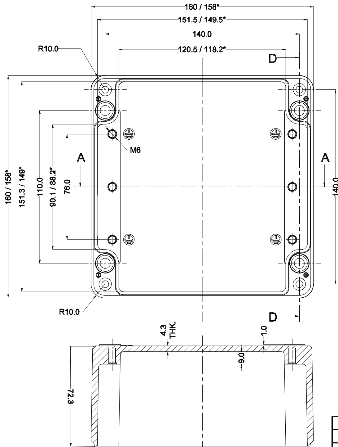
SECTION A-A
