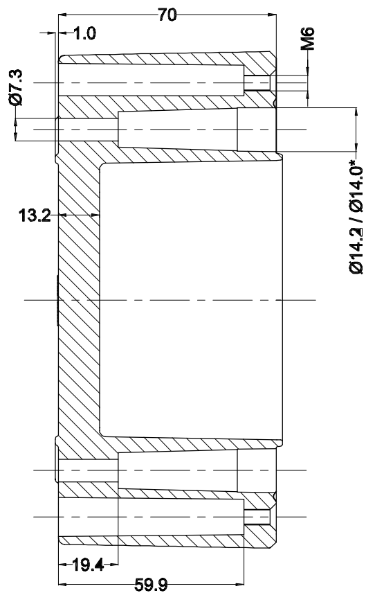
SECTION D-D
