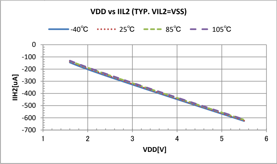
V DD VS I I L2 (TYP. V I L2=VSS)
