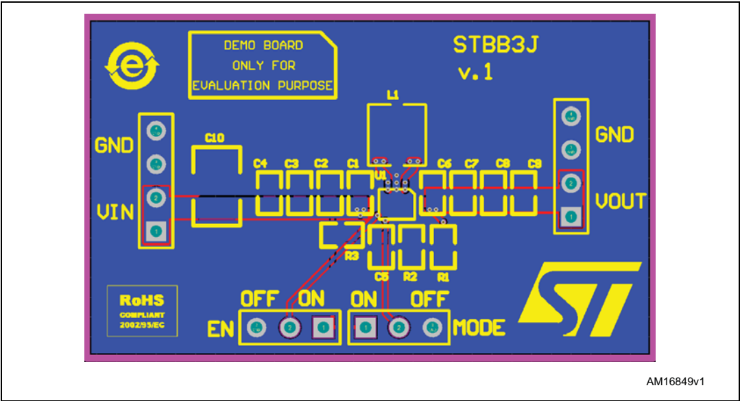
Figure 34. Bottom layer
