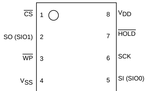
UDFN8 (LE25S161PCTXG)
