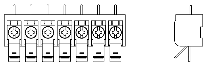
9-1437651-3 .250 TYP
