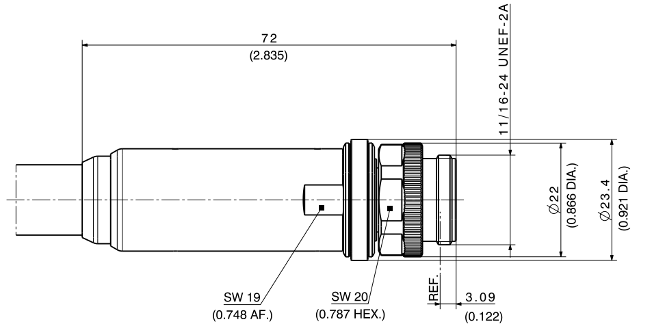
35 VM (3.5 mm ruggedized DUT male)
