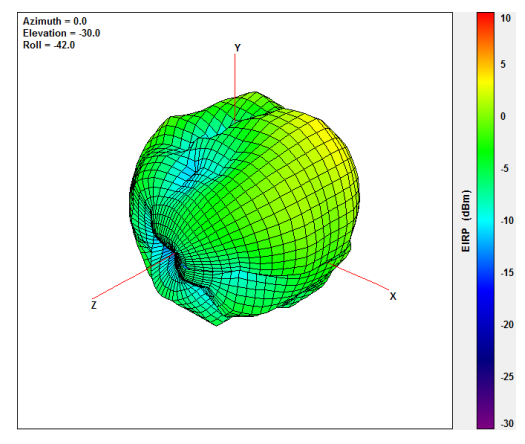
@1880MHz
