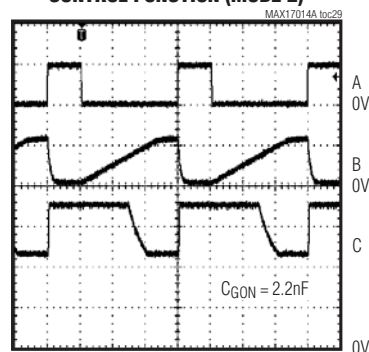
A: V_{CTL} , 5V/div B: V_{MODE} , 2V/div C: V_{GON} , 10V/div
