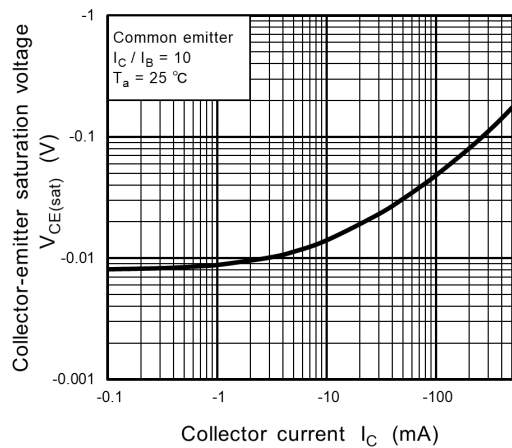
Fig. 6.3 V_{CE(sat)} - I_C
