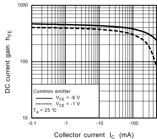
Fig. 6.2 h_{FE} - I_C
