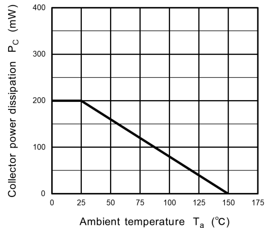
Fig. 6.4 P_C - T_a
