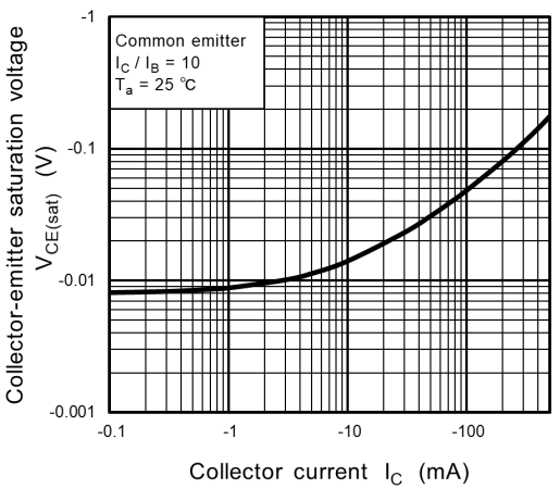
Fig. 6.3 V_{CE(sat)} - I_C
