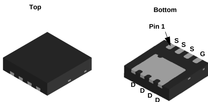
MLP 3.3x3.3
