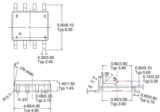
(4) SOP-8L
