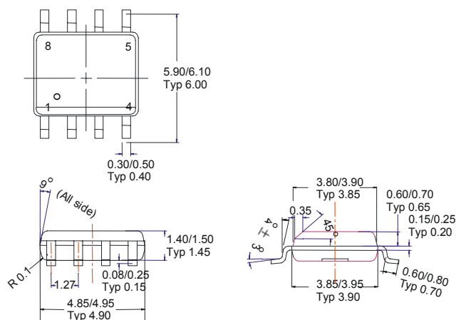
(4) SOP-8L
