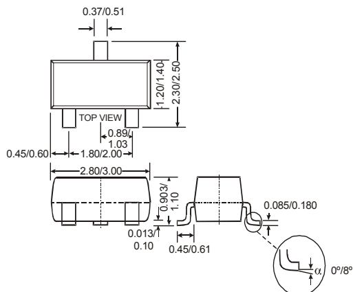
(3) SOT23(R)
