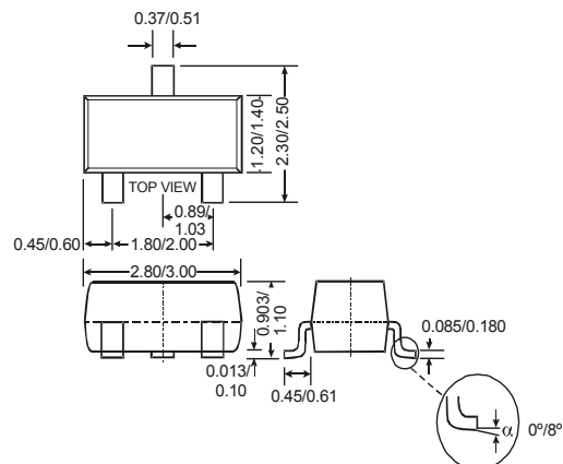
(3) SOT23(R)
