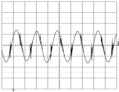
Trace: output voltage (20 mV/div.). Time scale: (2 μs/div.).
