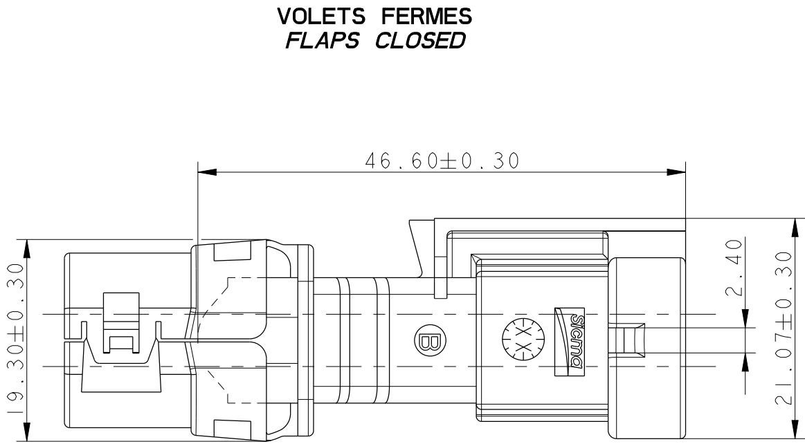
VOILETS OUVERTS POSITION DE LIVRAISON FLAPS OPENED DELIVERY POSITION
