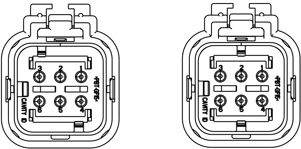
2098238-2 PURPLE TPA KEY B SCALE 2:1 2098238-3 BLUE TPA KEY C SCALE 2:1
