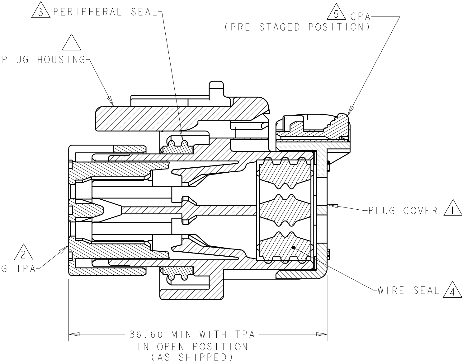
SECTION A-A
