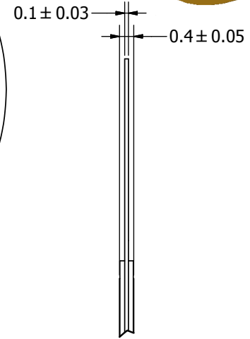
A ( 10 : 1 )
