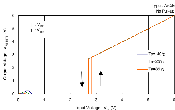
XC6129C ( V_{DF(T)} \approx 2.7V )
