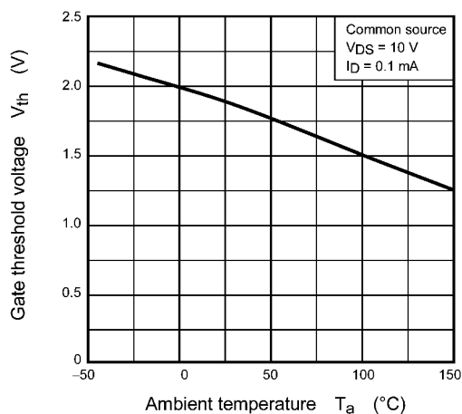
Fig. 7.7 V_{th} - T_a
