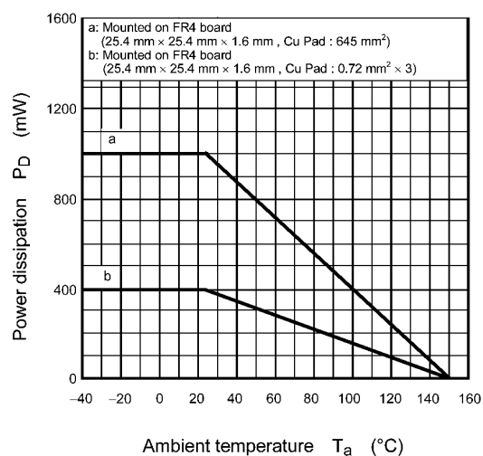
Fig. 7.14 P_D - T_a
