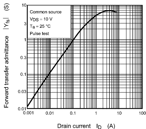
Fig. 7.8 |Y_{fs}| - I_D
