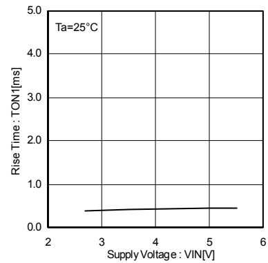
Fig.19 Output rise time
