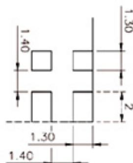
A-A 視圖 SCALE:4:1
