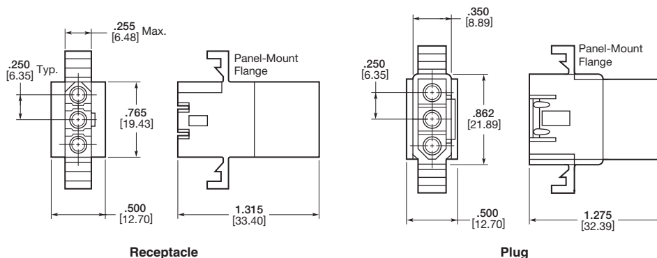
Receptacle
