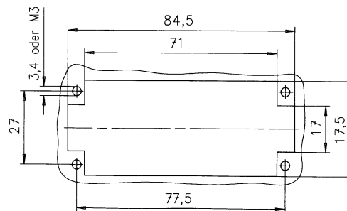
Montageausschnitt (Kontaktträger) Panel cut out (insert)
