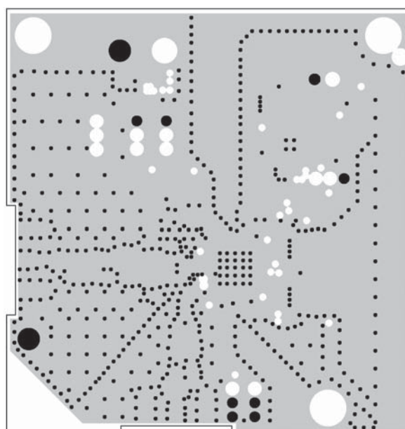
Inner Layer 3
