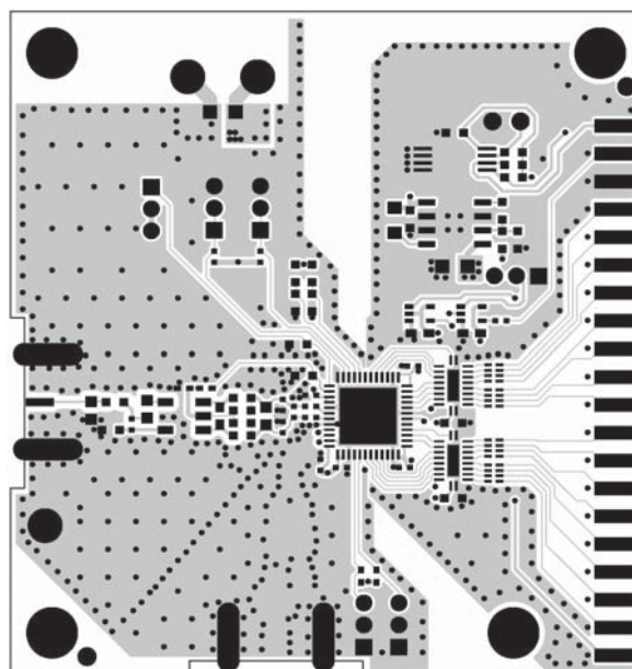
Top Side
