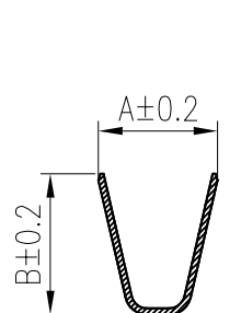
SEC A-A
